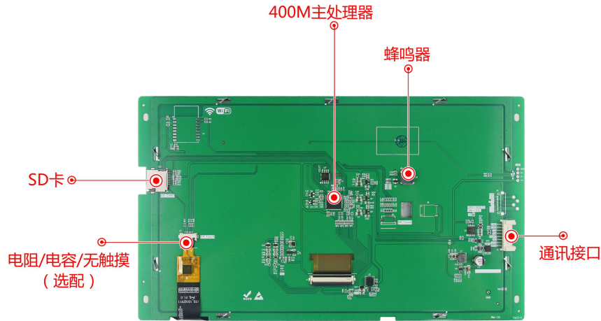
图 1-4 硬件配置图
