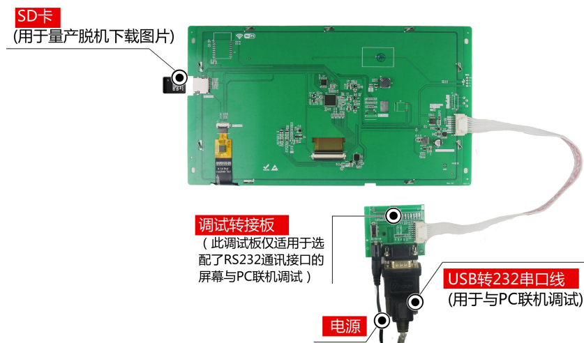
图 1-5 调试工具图
